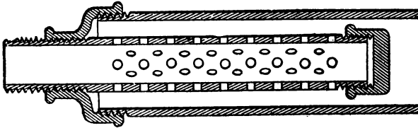
FIG. 17.—Gas Pipe Muffler.
